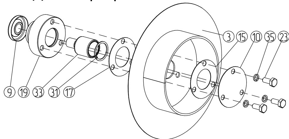
Диск маркера
