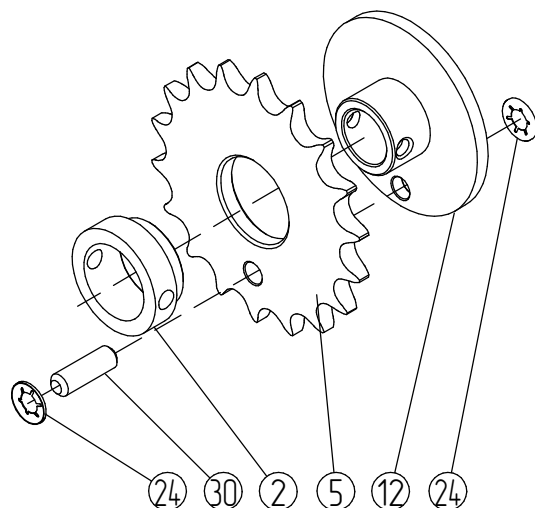
Муфта предохранительная
