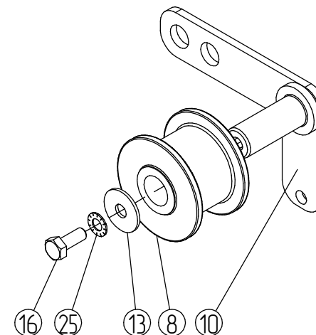
Осевой натяжек
