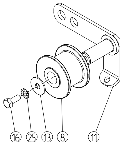
Звездочка 15-15,875
