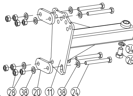
Кронштейн диска
